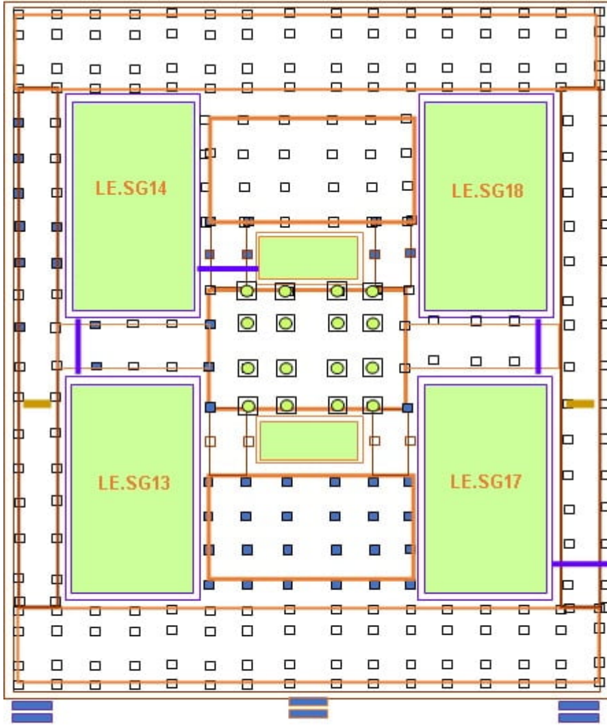
Phục dựng kết cấu mặt bằng khu kiến trúc trung tâm chùa Quỳnh Lâm thế kỷ 18 do chúa Trịnh Giang cho xây dựng theo tư liệu Khảo cổ học
