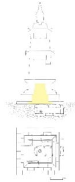
Cấu trúc tháp chùa Đá Chồng, Đông Triều, Quảng Ninh) Nguồn: Nguyễn Ngọc Tân
